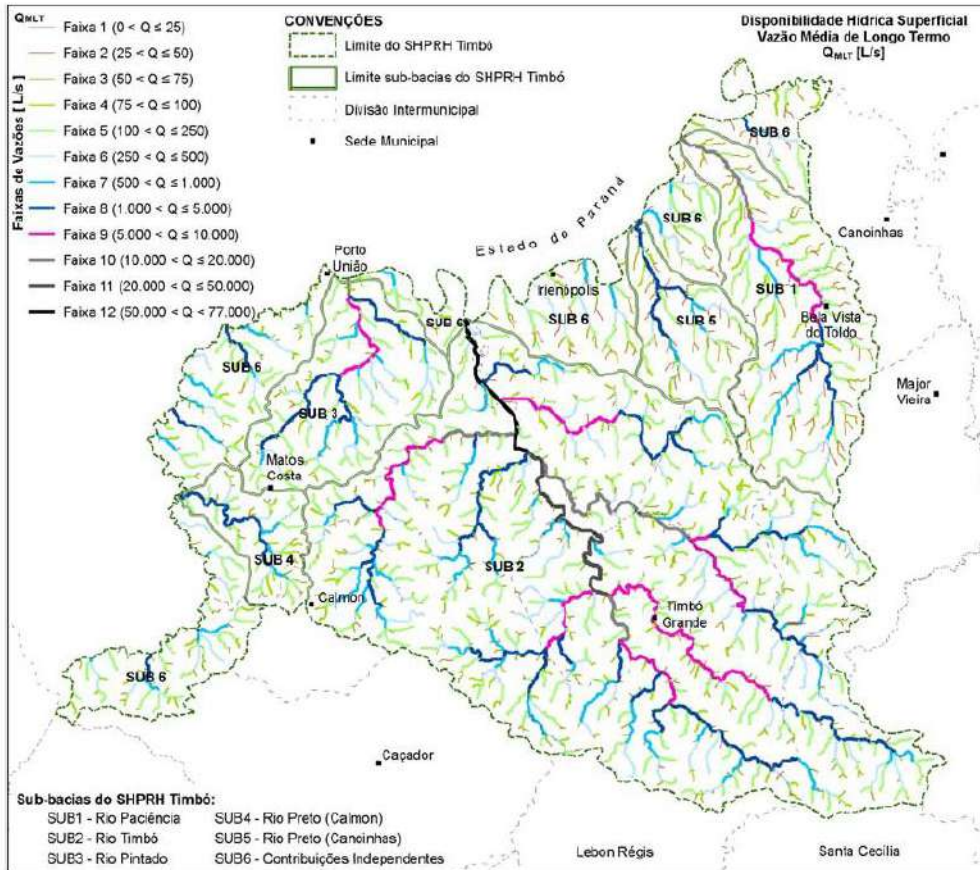
Figura 38 – Disponibilidade Hídrica 2009 – Qmlt do SHPRH Timbó.
