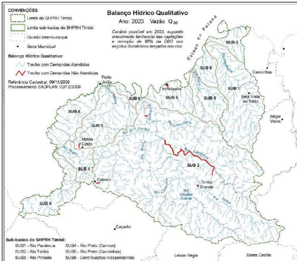
Figura 53 – Balanço Hídrico Qualitativo Q98: 2023 – Saída SADPLAN – Cenário 1.
