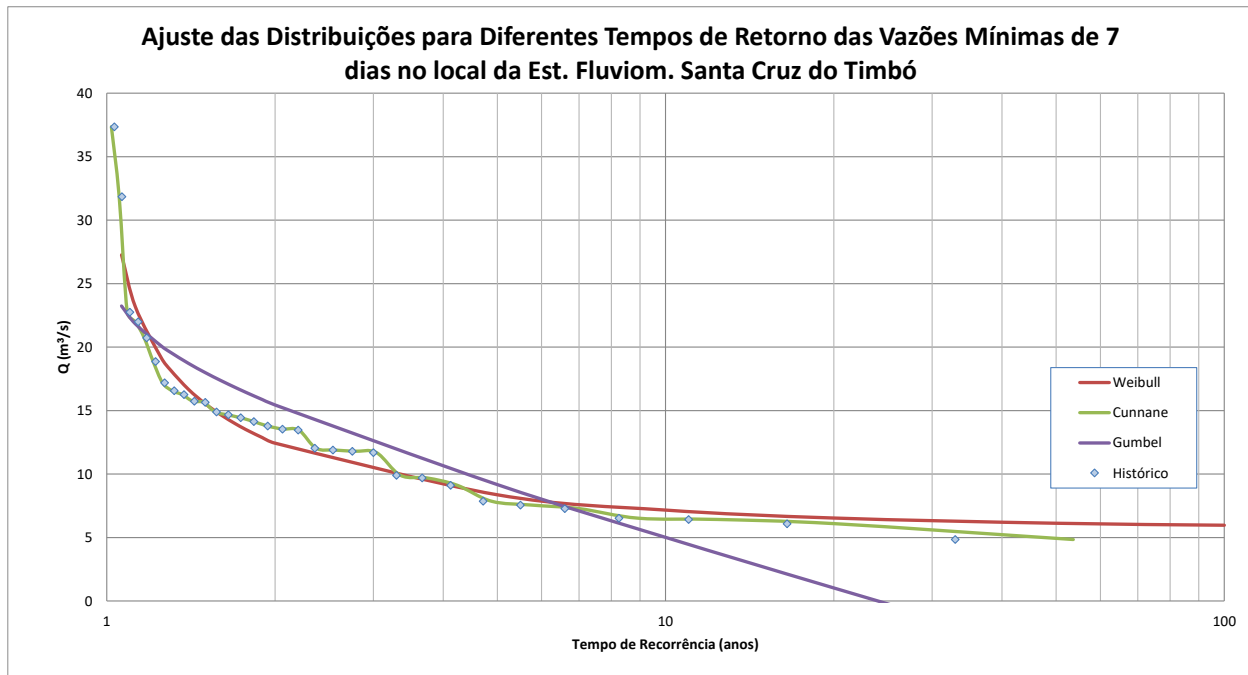
Figura 29 - Ajuste das Distribuições Para Diferentes Tempos de Retorno das Vazões Mínimas Médias de 7 dias Consecutivos – E. F. Santa Cruz do Timbó.
