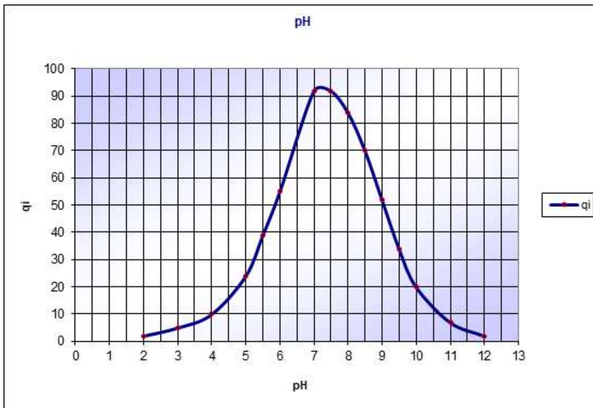
Figura 60 – pH – IQA.
