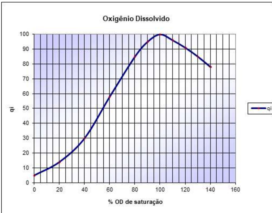
Figura 58 - % de OD – IQA.
