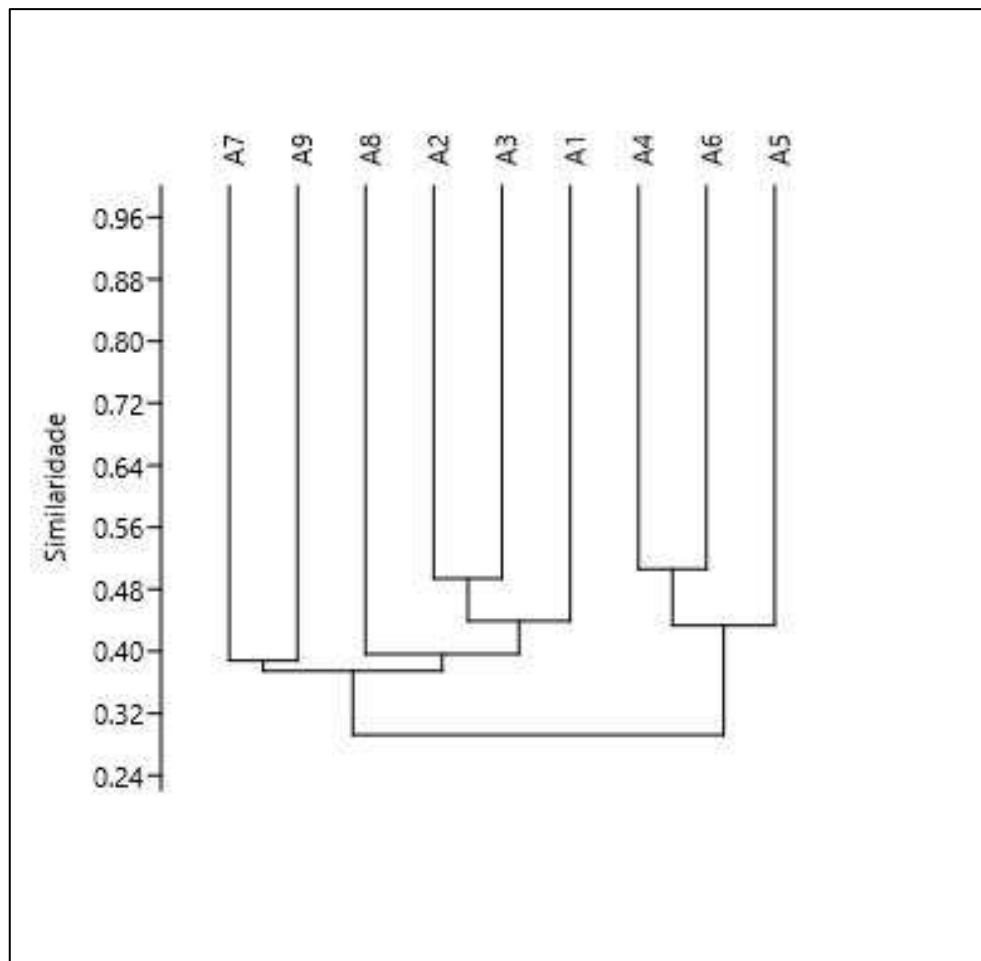
Figura 148 – Dendrograma de similaridade da avifauna nos pontos fixos nas áreas amostrais na Bacia do Rio Tamanduá.
