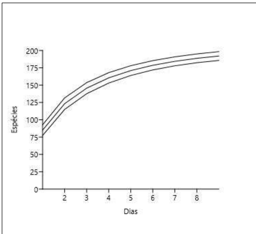
Figura 141 – Curva de rarefação das espécies da avifauna registradas nas áreas amostrais da Bacia do Rio Tamandúá.
