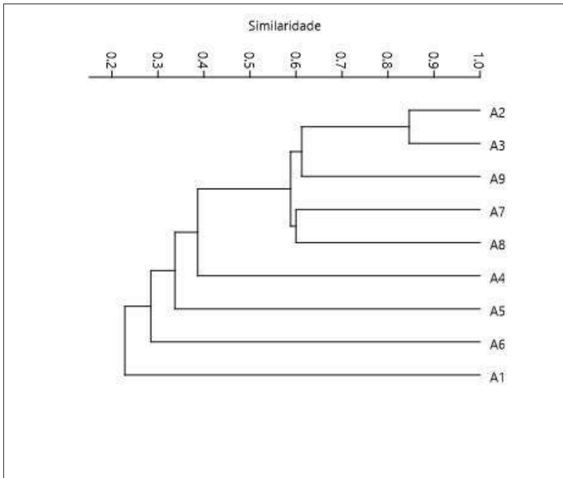
Gráfico 13 – Dendrograma de similaridade gerado através do índice de Jaccard comparando as áreas amostrais na Bacia do Rio Tamandúá.
