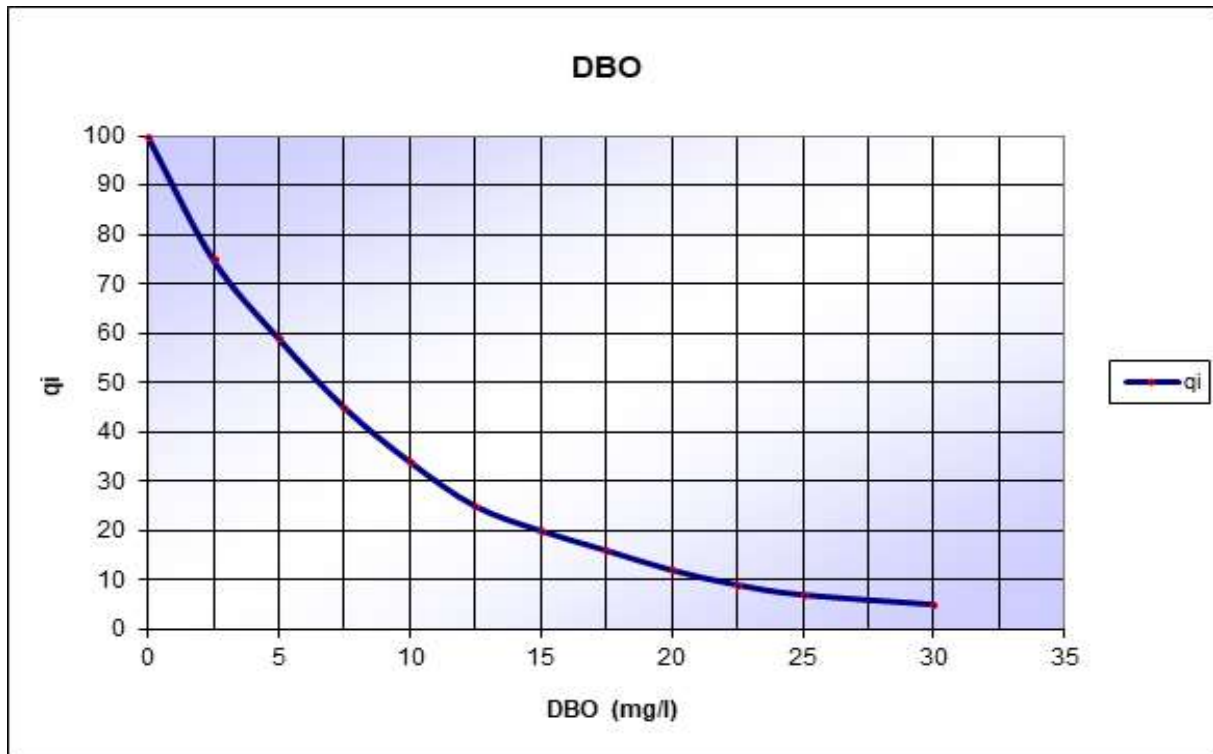
Figura 61 – DBO – IQA.
