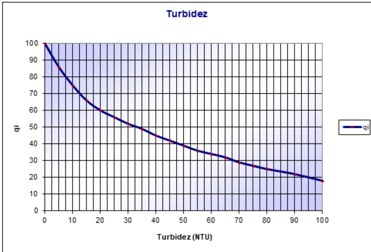
Figura 65 – Turbidez – IQA.
