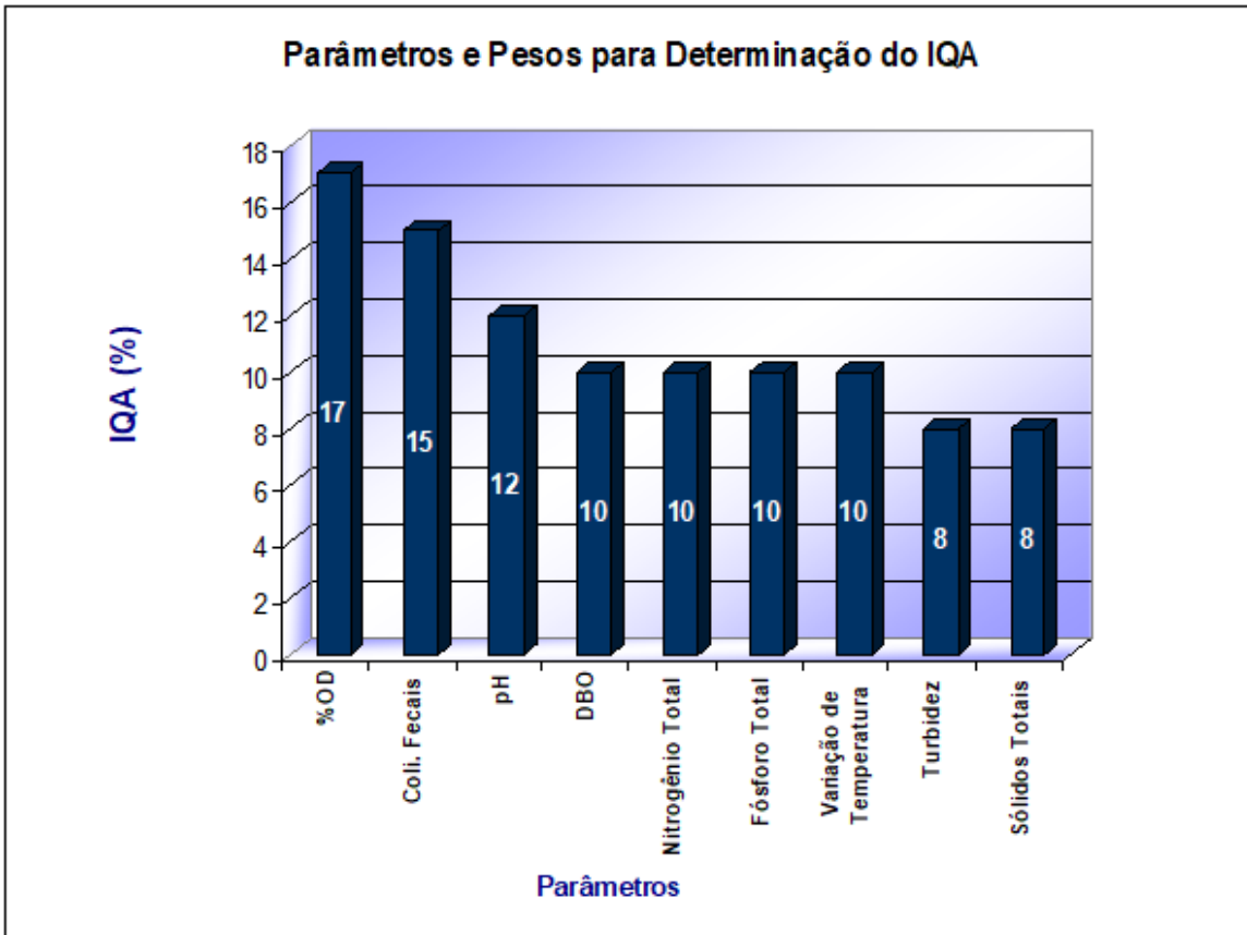
Figura 57 – Pesos dos Parâmetros do IQA.
