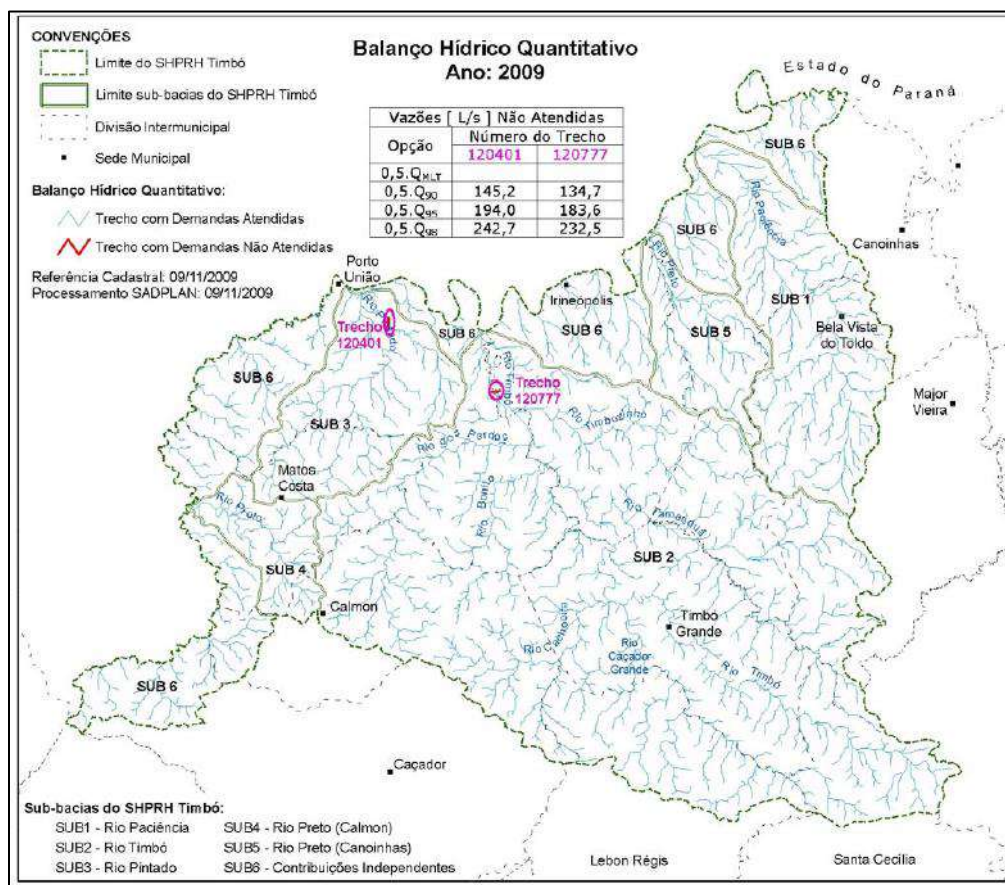
Figura 45 – Balanço Hídrico Quantitativo: 2009 – Saída SADPLAN.
